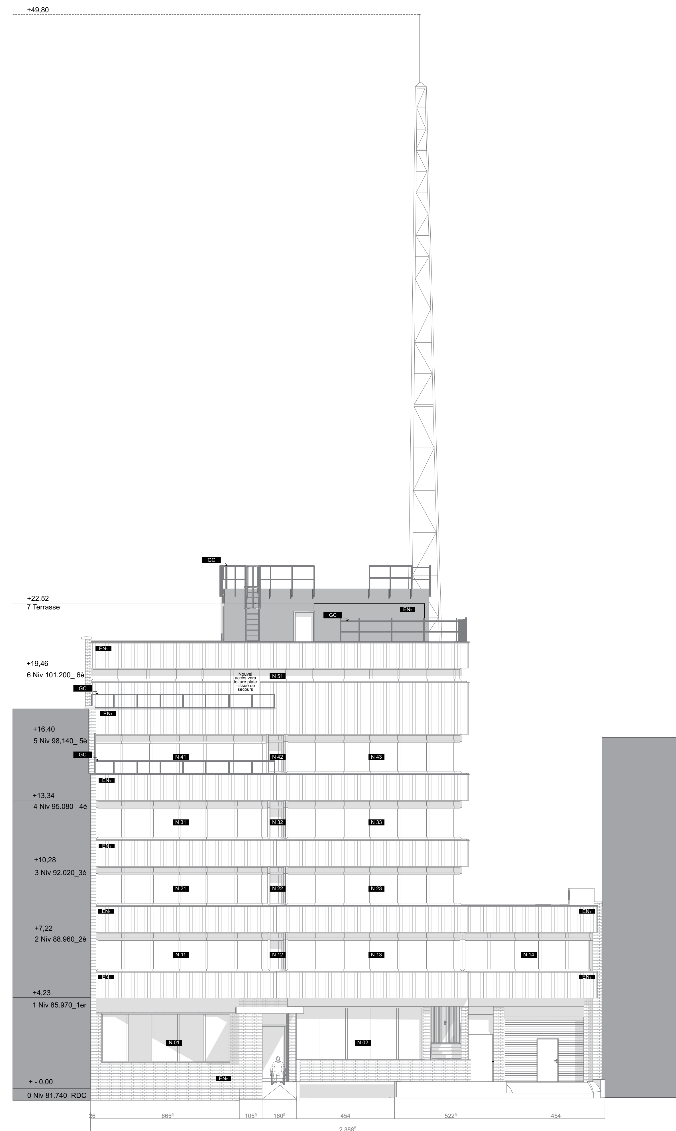
Façade nord - Noord gevel
