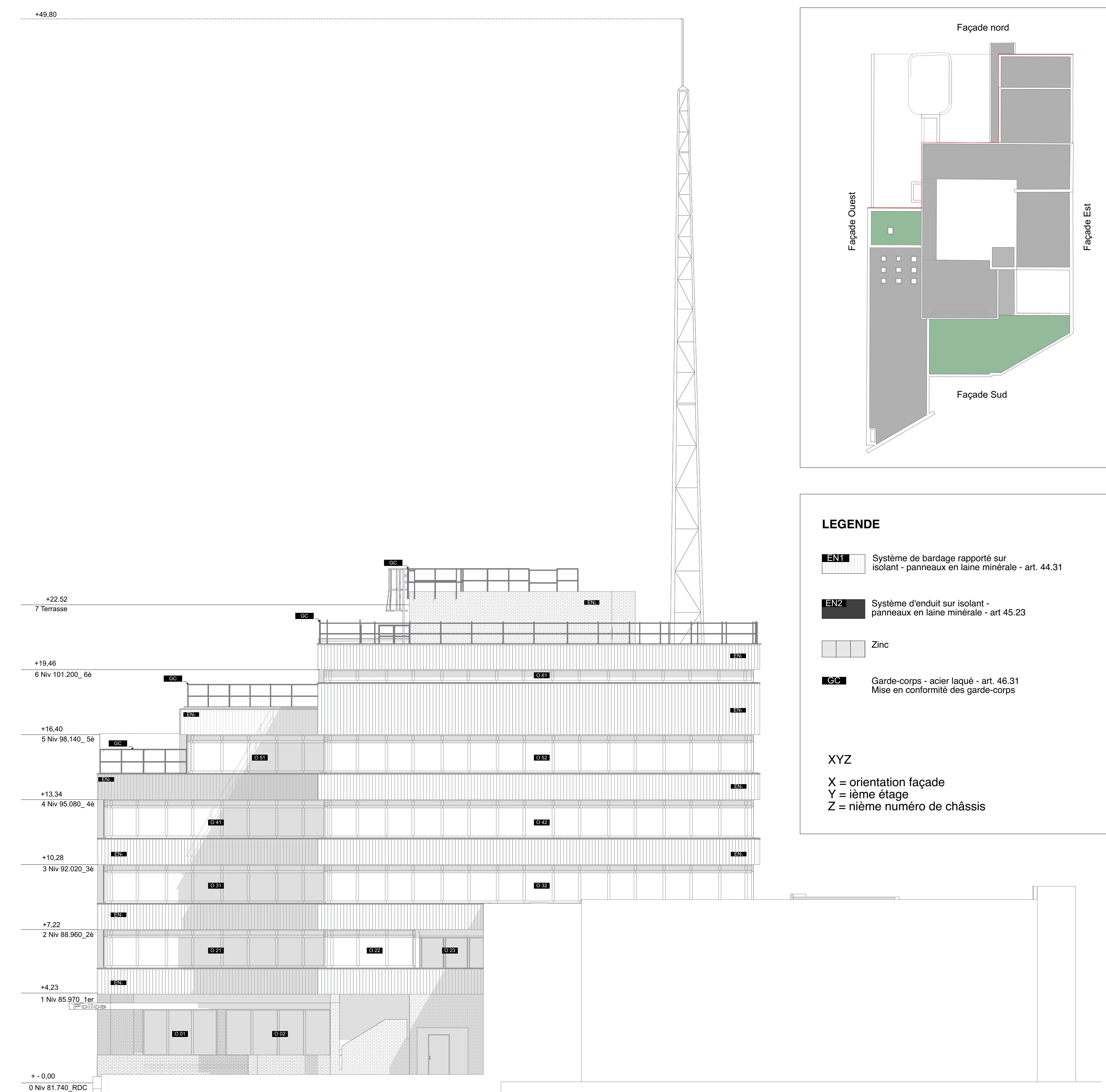
Façade ouest - Oost gevel
